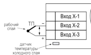
Рисунок 5.18 – Схема подключения термопары
