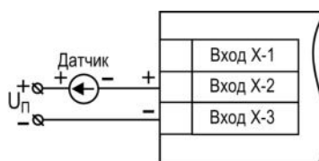
Рисунок 5.21 – Схема подключения пассивного датчика с токовым выходом 0\dots5 мА или (4)\dots20 мА
