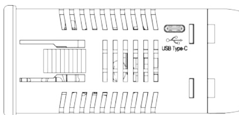
Рисунок 5.10 – Расположение разъема USB для корпуса Ц5
