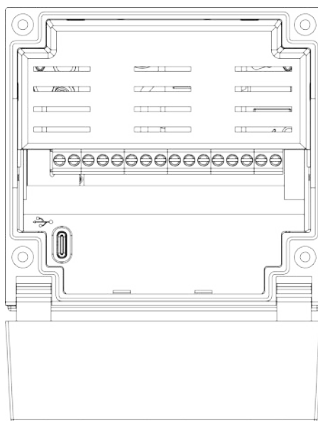
Рисунок 5.12 – Расположение разъема USB для корпуса H
