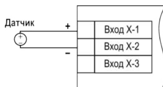
Рисунок 5.20 – Схема подключения активного датчика с выходом в виде напряжения 0\dots5 В и 0\dots10 В
