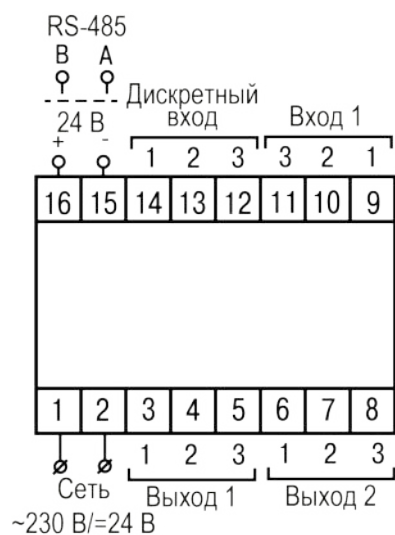
Рисунок 5.6 – Общая схема подключения TRM10–Д
