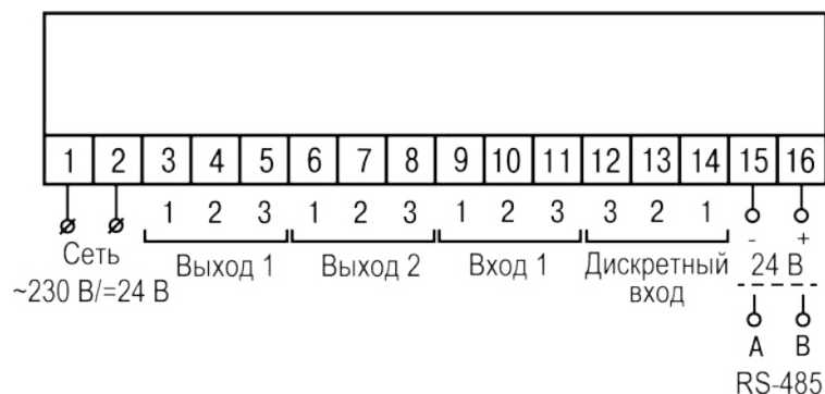
Рисунок 5.4 – Общая схема подключения TRM10–Щ1/Щ2
